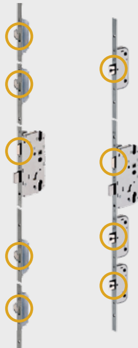
VARIANTE 1: Mehrfachverriegelung (5-fach) mit 4 Schließhaken VARIANTE 2: automatische Mehrfachverriegelung (4-fach) mit 3 automatischen Fallenriegeln ( autolock )
