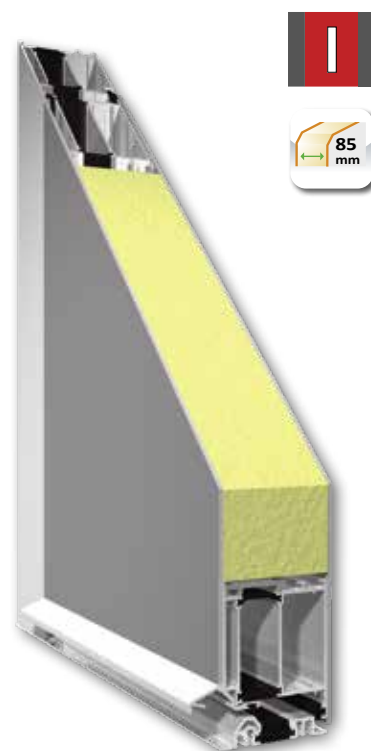
Türblatt: ALUMINIUM beidseitig flügelüberdeckend
