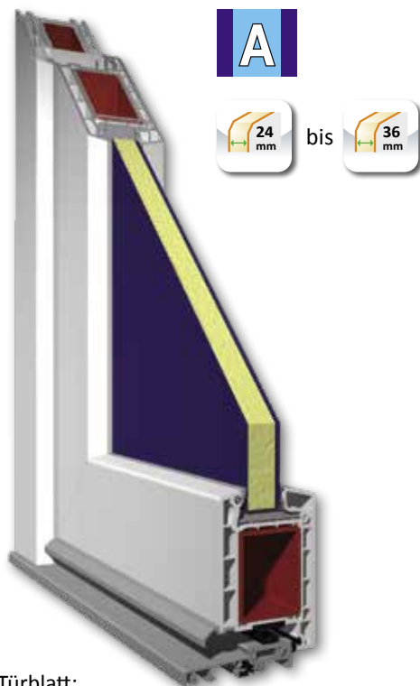
Türblatt: KUNSTSTOFF GFK
