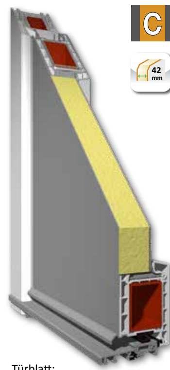
Türblatt: ALUMINIUM einseitig flügelüberdeckend
