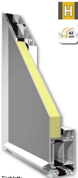
Türblatt: ALUMINIUM eins. flügelüberdeckend
